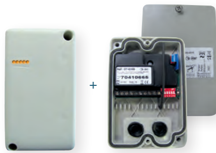
1 GPRS-Modul
